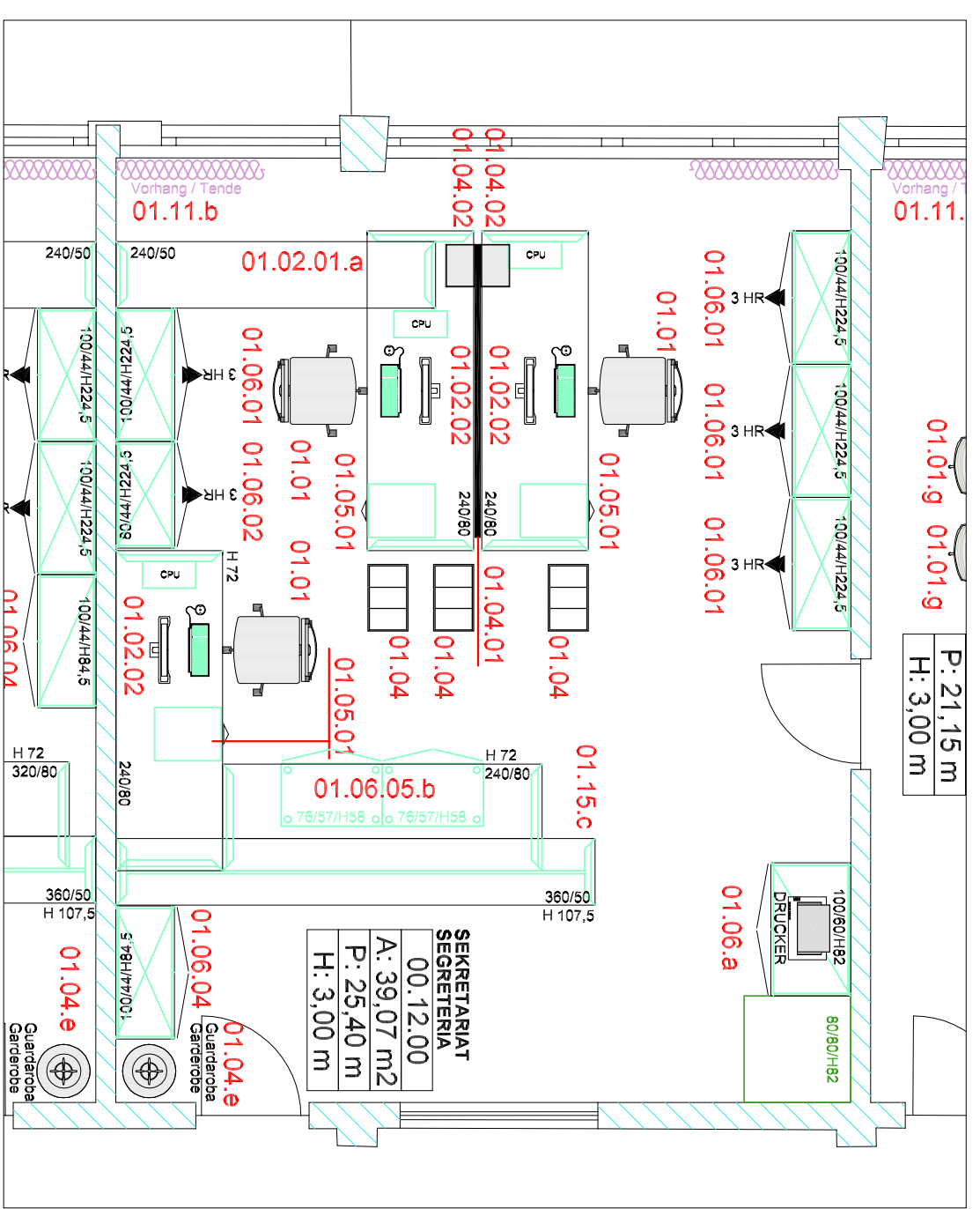
PIANO TERRA - ARREDAMENTO 1: 50 ERDGESCHOSS - EINRICHTUNG 1: 50
